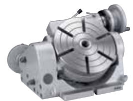
Schwenkbarer Rundtisch TSK
