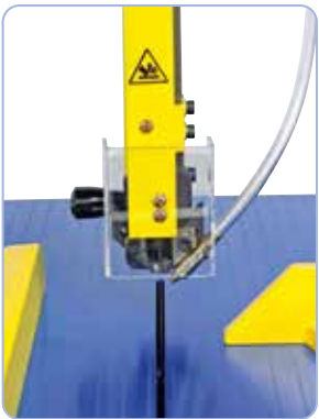
Inclusief uitblaasinrichting voor optimaal zicht op de zaaglijn
