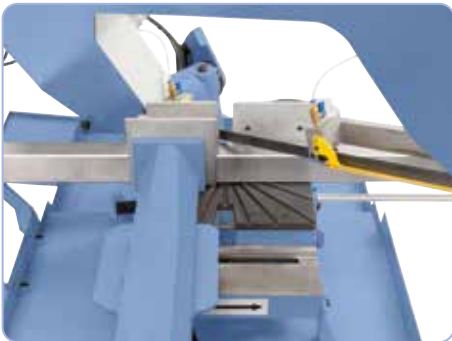
Materiaalklem met snelklemming voor dubbelverstekzagen verschuifbaar
