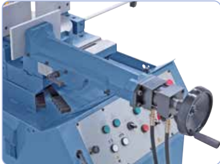
Verschuifbare materiaalklem, klemming gebeurt manueel of hydraulisch
