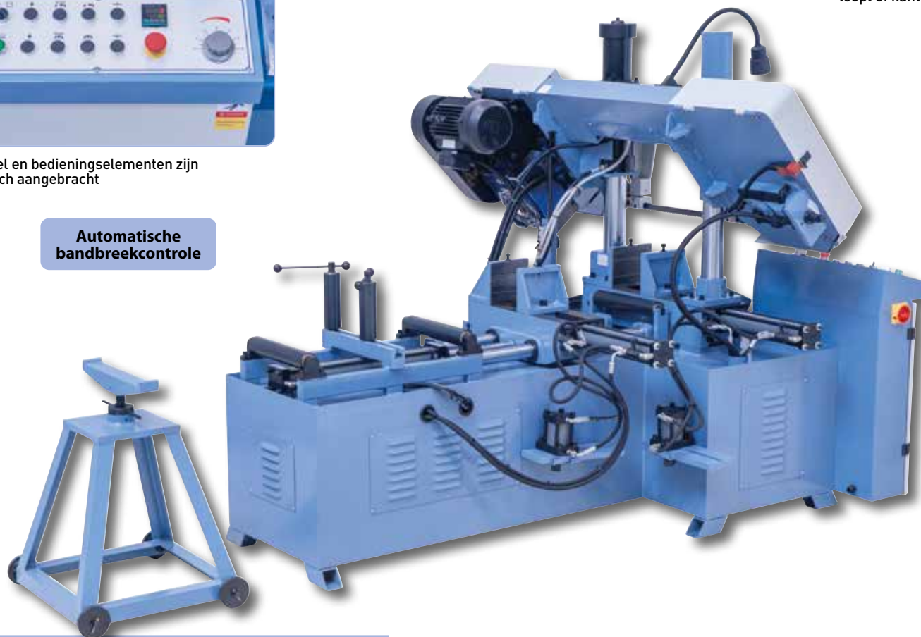
De verstelbare zaagbladgeleider voorkomt dat het zaagblad zijwaarts loopt of kantelt.
