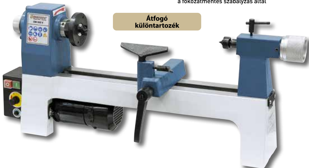
Alapfelszereltségben 110 mm, ill. 175 mm késtámasszal.
