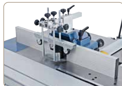
A maró-védősapka eloxált alumínium ütközősínekkel felszerelt
