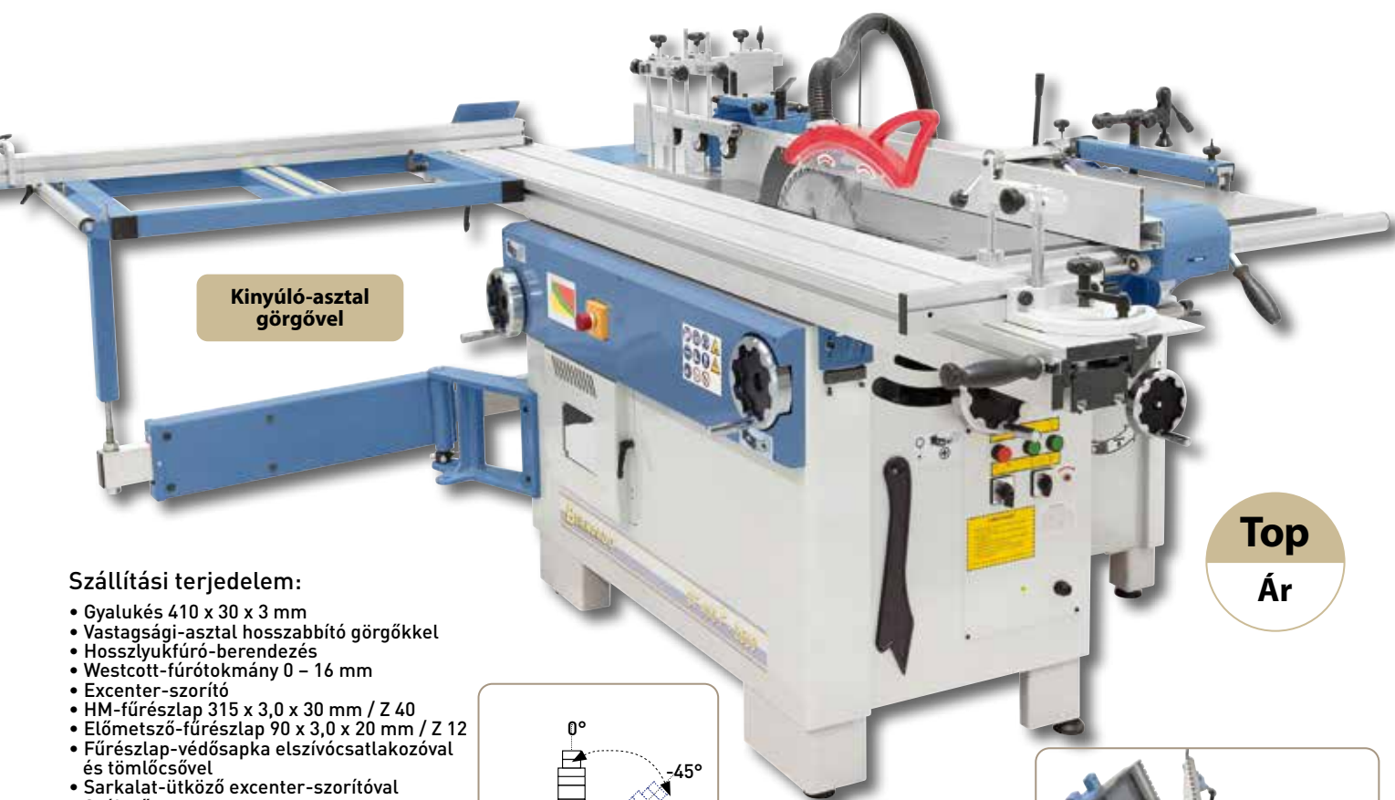
A fűrészlapvédő integrált elszívő-csatlakozóval a hasítóéken van rögzítve. Sorozatszerűen előmetsző-aggregáttal felszerelve
