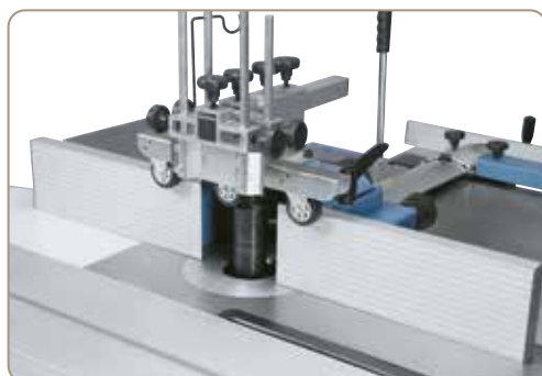
Masszív maró-védősapka finoman beállítható ütközősínekkel
