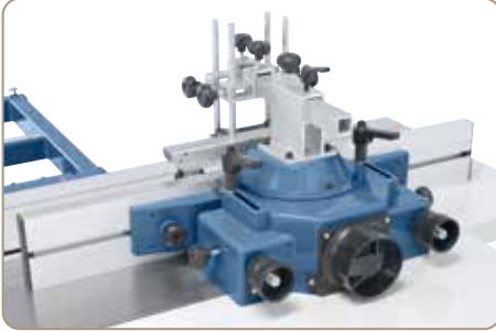
A maró-védősapka finom-beállítással felszerelt. A forgács elvezetése integrált elszívó-csatlakozón keresztül történik.
