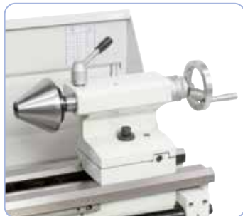
Takapyökkä pikalukituksella. Lisävarusteena saatavilla keskityskartio.
