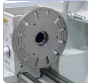
Erityismuotoisten työkalupaleiden kiinnittämiseksi voidaan koneeseen asentaa kiinnitysliukka 250 mm.
