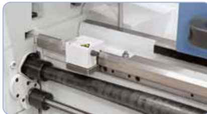
Vakiona mikrometri pitkittäisvasteessa ja johtoruuvin suojus.
