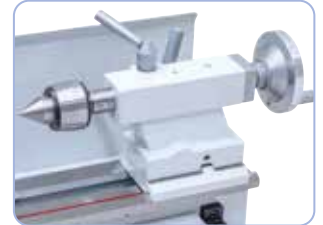
Takapyykkä, jossa MK 2 kiinnitys, voidaan muuttaa kartiosorvaamista varten
