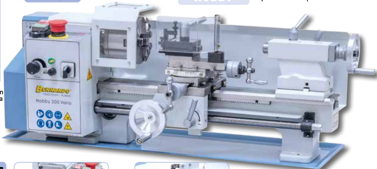
Koneessa on vakiona pikavaihtoteränpidin
