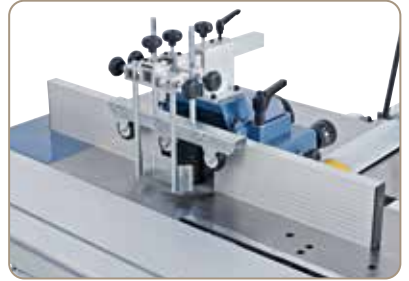
Fræserbeskyttelsesskærmen er udstyret med eloxerede aluminium-anslagskinner.
