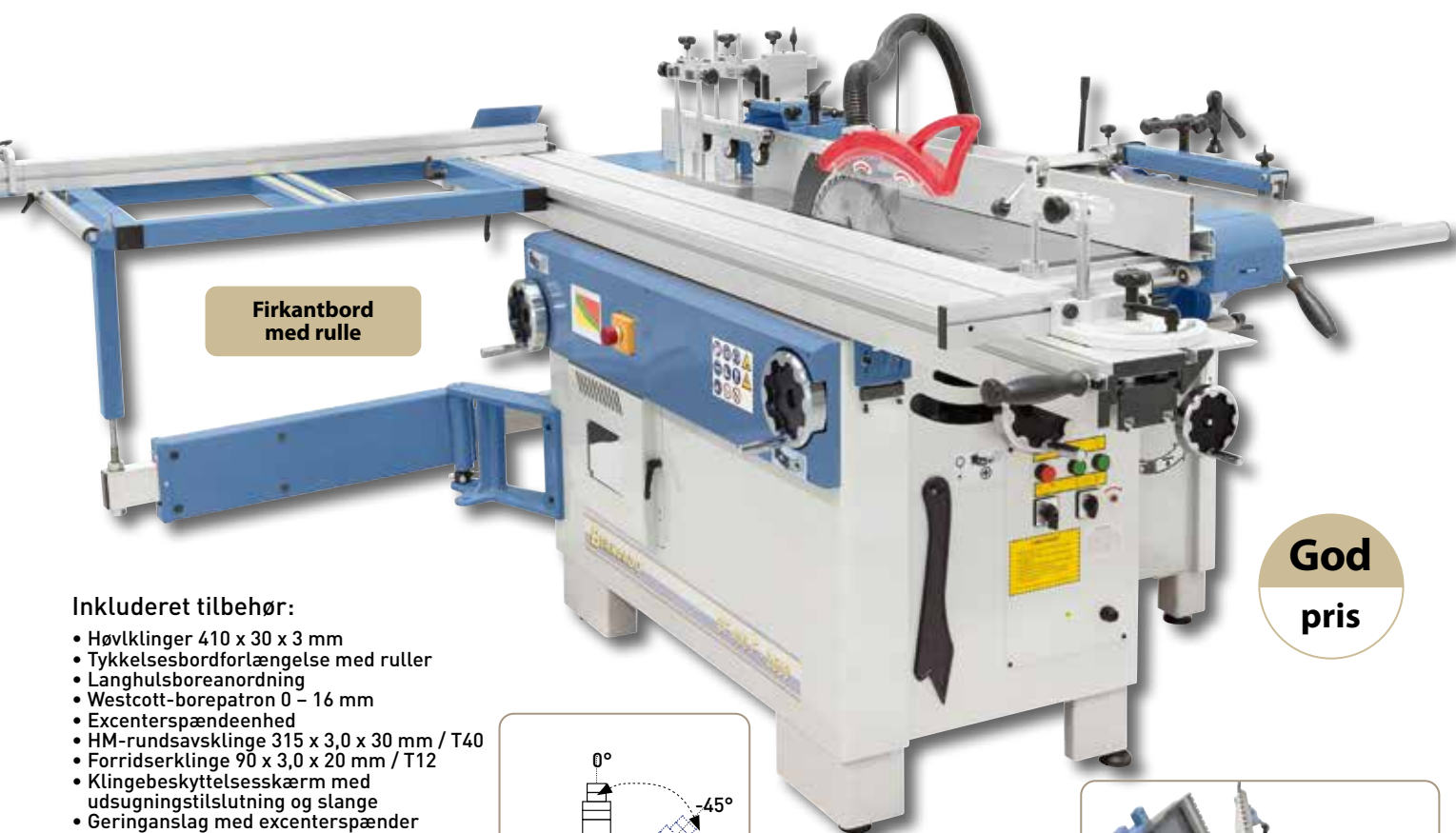
Fræserbeskyttelsesskærmens anslag kan indstilles hurtigt og enkelt til det pågældende fræseværktøj. Den standardmæssige beskyttelsesanordning forhindrer, at emnet føres tilbage.
