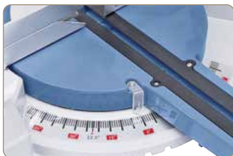
Stabil drejeskive med integreret gradskala, til geringsnit, kan svinges 45° til venstre og højre.
