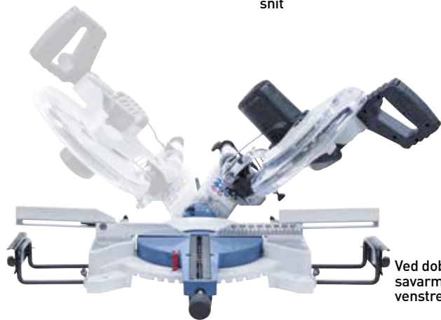
Udtrækkelig bordudvidelse i begge sider med pålægningsflade og opklappelige anslag til gentagende snit
