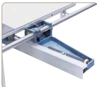
Ved skæring af store dele svinges parallelanslaget ganske enkelt af.
